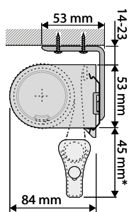
Fixation sur équerres
