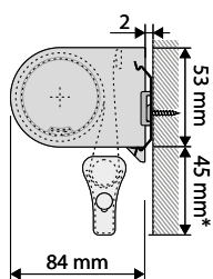
Fixation avec clips de montage (standard)
